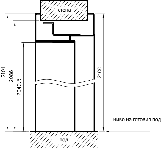
Вертикален разрез OSRB
