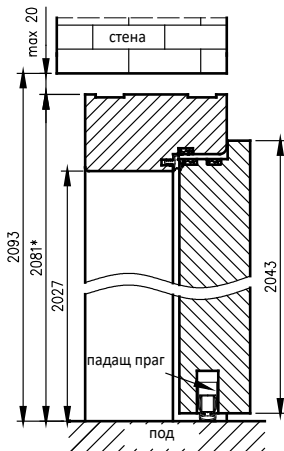
Дървена каса за врати Athos с падащ праг*
