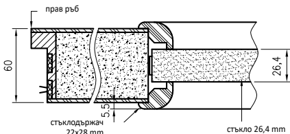
Пожароустойчиво крило Olimp EI60
