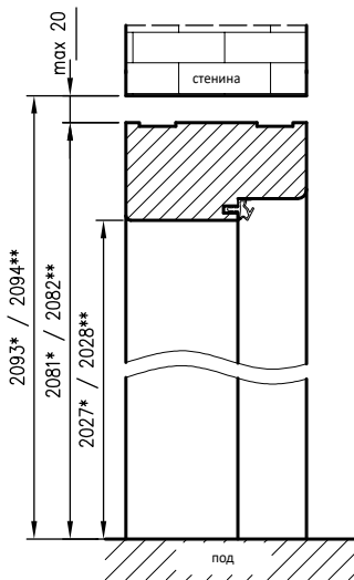
Вертикален разрез на пожароустойчива врата
