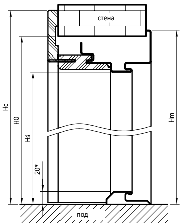
Размери OSH STAND за двукрили врати
