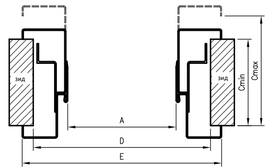
Хоризонтален разрез OSRB
