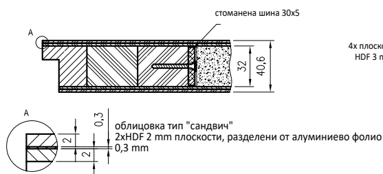
Блиндирани крила за врати Solid RC2
