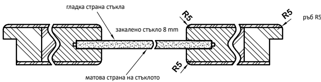
Хоризонтален разрез врати Vetro D1
