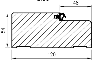
Разрез на дървена каса за врати OLIMP EI60
