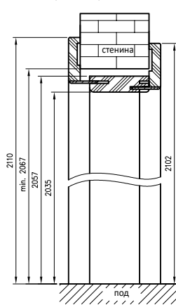
Вертикальный разрез на регулируемом туннеле с перемычкой Т63
