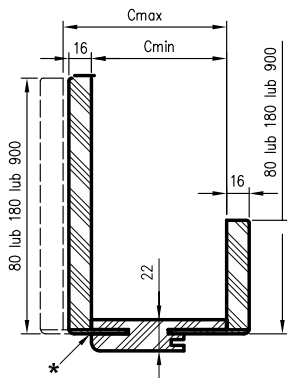
Разрез на гредата
