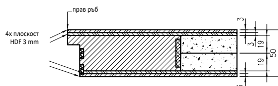
Пожароустойчиви крила за врати Athos EI30
