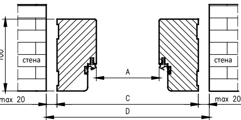
Размери OD за врати Athos
