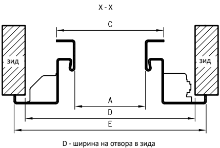
размери за еднокрили врати
