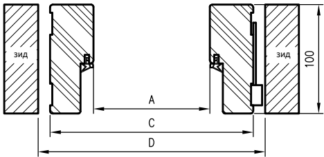
Хоризонтален разрез OPB
