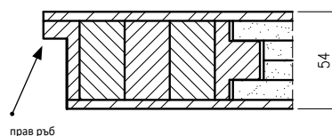
Блиндирано крило NEFRYT RC2/RC3
