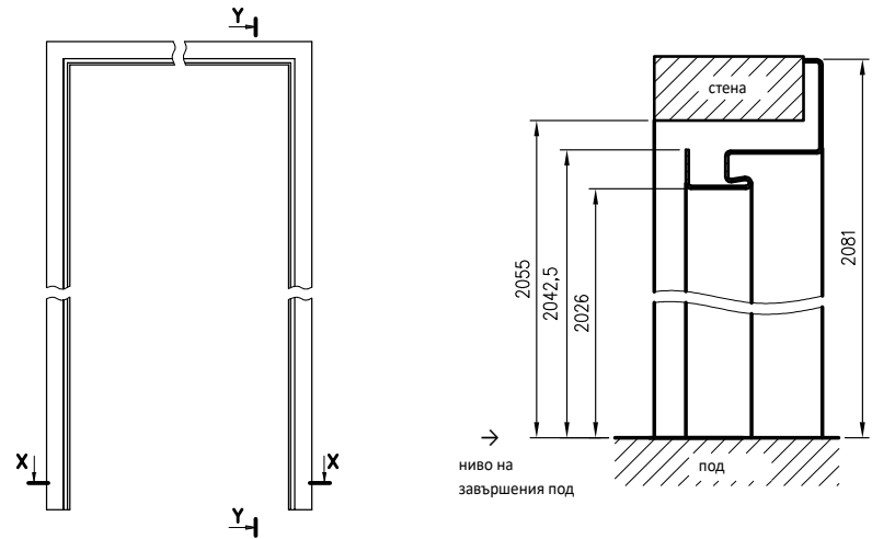
размери за еднокрили врати
