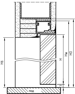
Профил DRE за безфалцови врати, отварящи се навън
