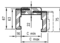
Разрез TUN с перемычкой Т63
