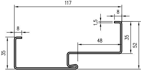
Профил на касата
