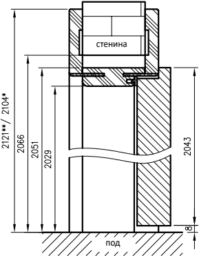
Вертикален разрез фалцови врати с OR
