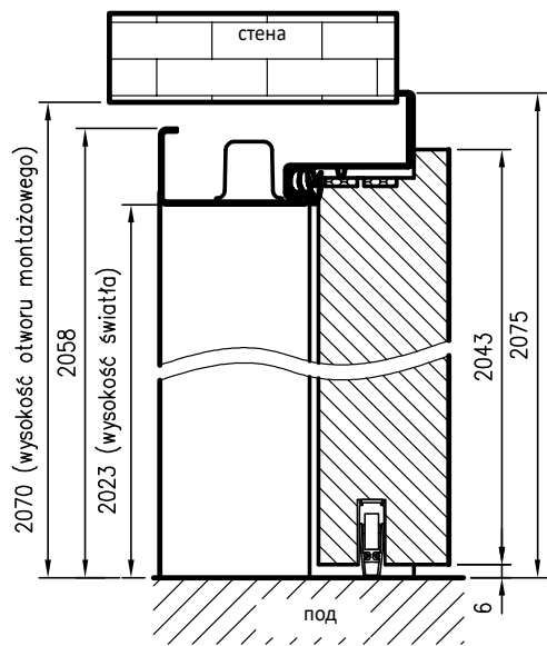
Размери Olimp EI60 за еднокрили врати
