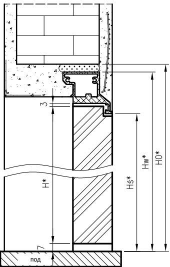
Профил DRE за врати, отваряеми навътре, с обратен фалц
