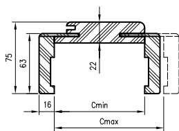
Разрез OR/ORC с перваз Т63
