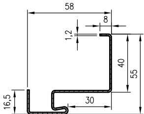
Профил на каса OSMK
