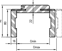
Разрез OR/ORC с перваз Т80
