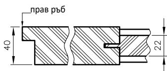
Хоризонтален разрез врати Nestor
