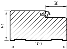
Разрез на дървена каса за врати OLIMP EI60
