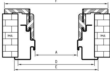
Профил на касата
