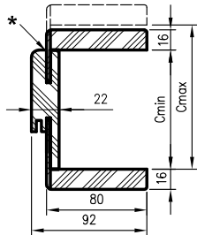
Разрез на гредата
