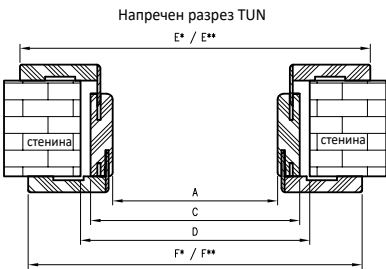
Разрез TUN с перемычкой Т80
