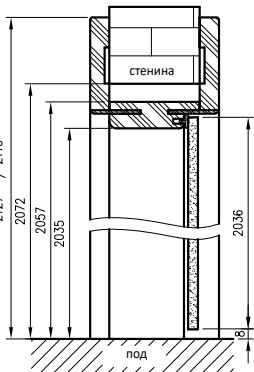
Вертикален разрез на стъклени врати с ORC
