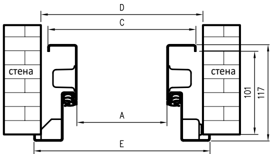
D - ширина на монтажния отвор
