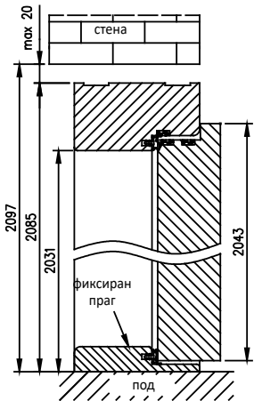
Дървена каса за врати Athos с фиксиран праг
