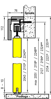
NS - вертикален разрез
