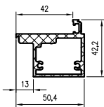
Профил DRE за безфалцови врати, отварящи се навън
