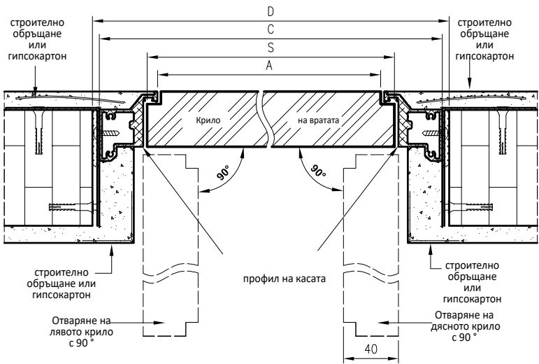
Размери ширина врати Sara Eco 2
