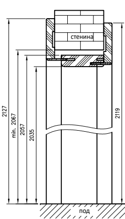
Вертикальный разрез на регулируемом туннеле с перемычкой Т80
