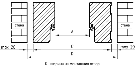
OD OLIMP EI30 за еднокрили врати
