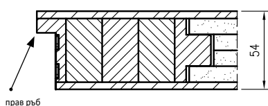
Блиндирано - пожароустойчиво крило NEFRYT RC2/RC3 EI-30
