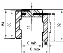
Разрез TUN с перемычкой Т63
