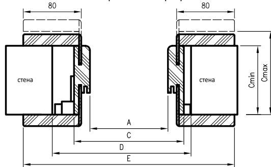
В-В Хоризонтален разрез
