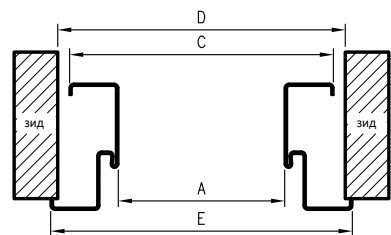
D - ширина на монтажния отвор
