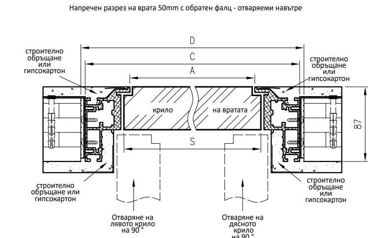
Размери ширина врати Profi
