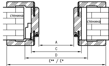
Хоризонтален разрез OR/ORC
