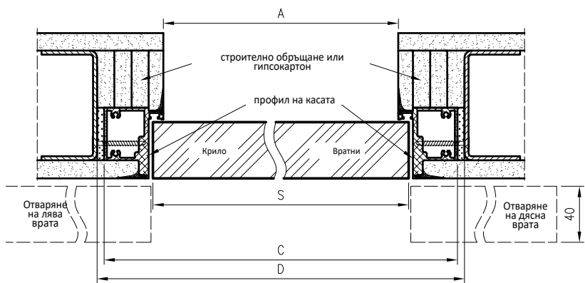
Размери ширина врати Sara Eco 2
